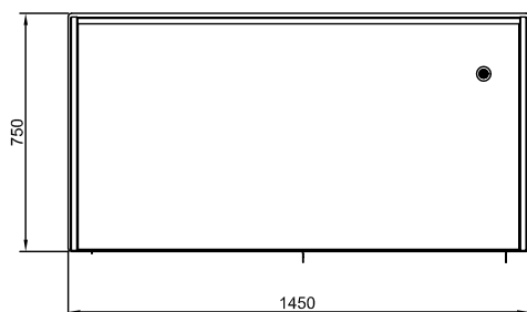
Boven aanzicht
