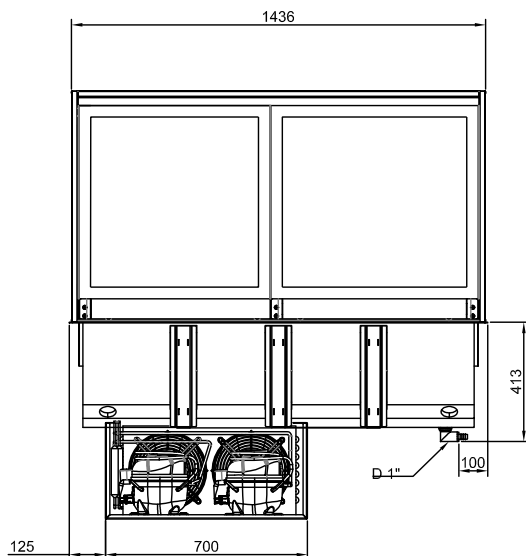
Zij aanzicht
